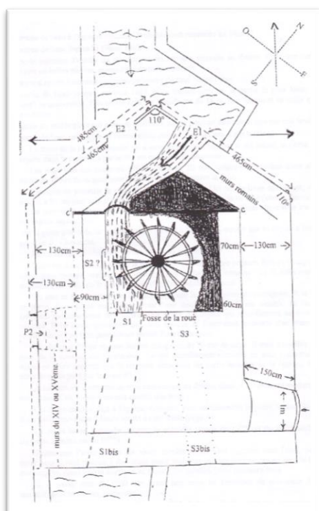
Partie médiévale du moulin du Belvezet (dessin H. Desparmet). L'arrivée du béal est en haut. La mention « murs romains » n'est pas fondée.
